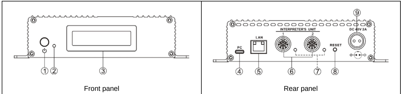
图 6.5.1 HCS-8685BM
